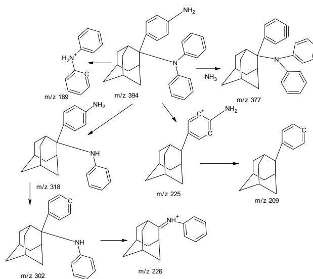
Рис. 1 Масс-спектр и схема масс-спектрометрического распада соединения 8
